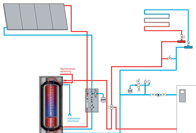
Wärmeerzeuger mit ThermoTank Quadroline Trinkwassererwärmer mit Solar, solare Erwärmung des Trinkwassers, Fußbodenheizung
