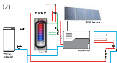
Einfache direkte Montage an einen Trinkwasserspeicher
