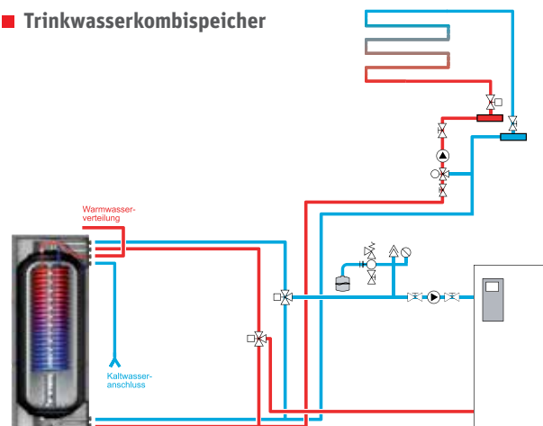
Wärmeerzeuger mit ThermoTank Quadroline Trinkwasserkombispeicher, Trinkwasserzone und Pufferzone, Fußbodenheizung
