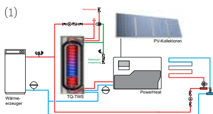
Einfache Montage an einen Trinkwasserspeicher mit integriertem Solarwärmetauscher
