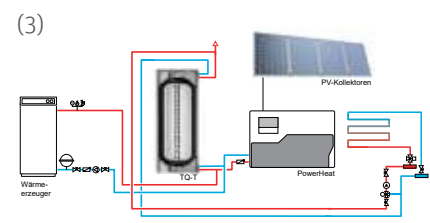
Einfache direkte Montage an einen Pufferspeicher
