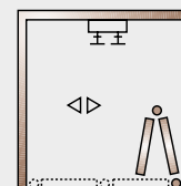
Einstiegsbreiten 845 x 845 = ca. 680 mm 745 x 745 = ca. 580 mm 795 x 845 = ca. 630 mm 945 x 945 = ca. 780 mm
