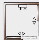
Einstiegsbreiten 845 x 845 = ca. 480 mm
